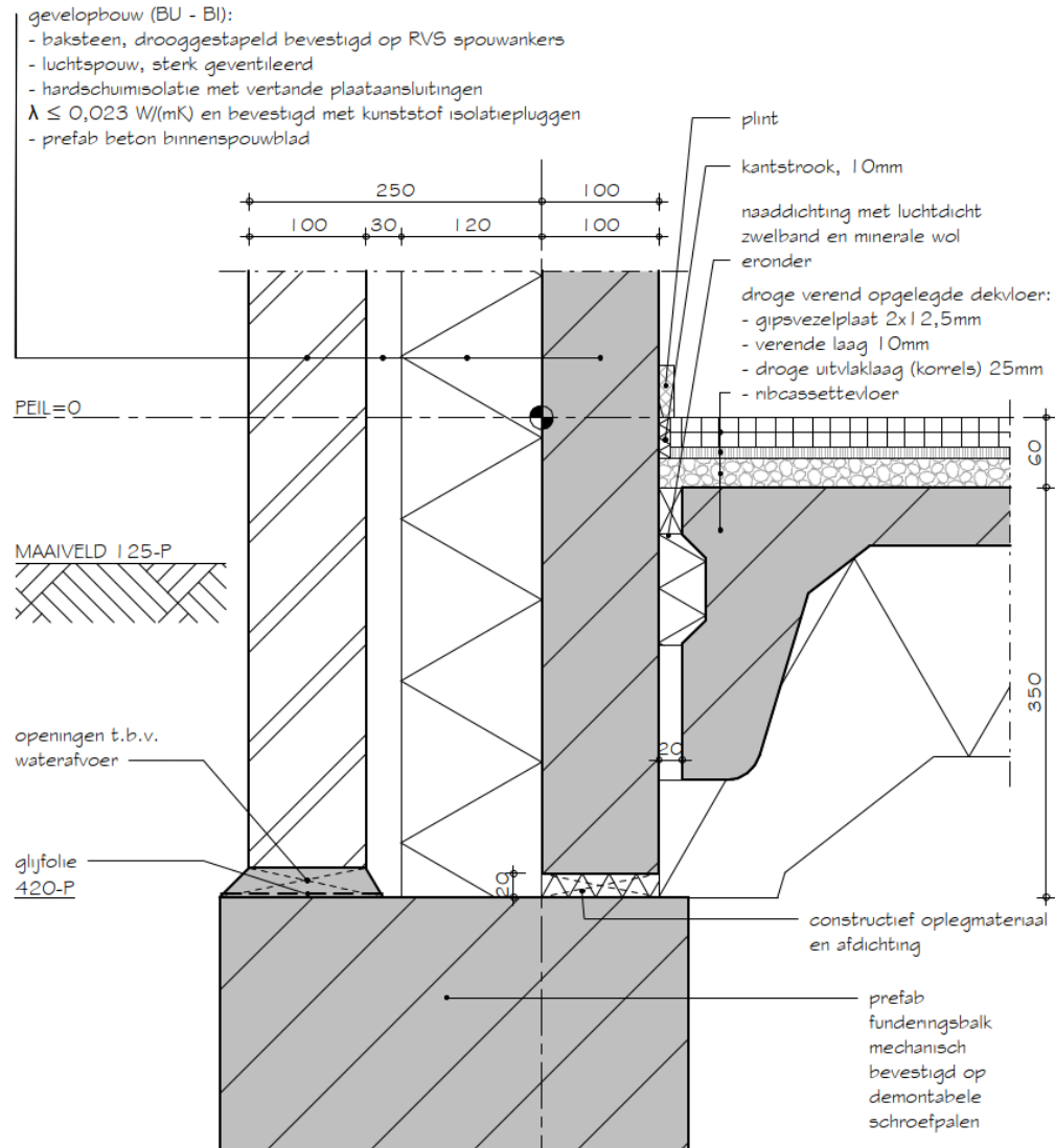
Figuur 8 – Dekvloer
