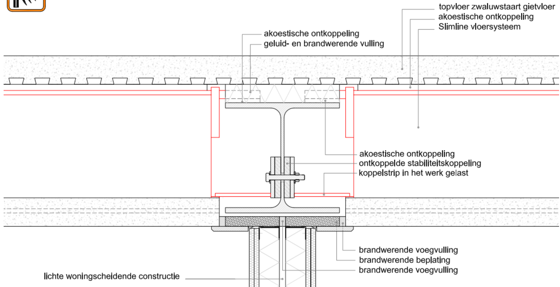
Figuur 20 – Staal-/prefabbetonvloer
